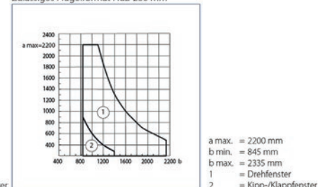
Zulässiges Flügelformat Hub 230 mm
