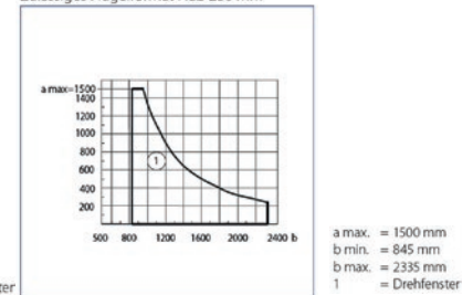
Zulässiges Flügelformat Hub 230 mm
