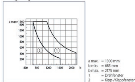
Zulässiges Flügelformat Hub 150 mm
