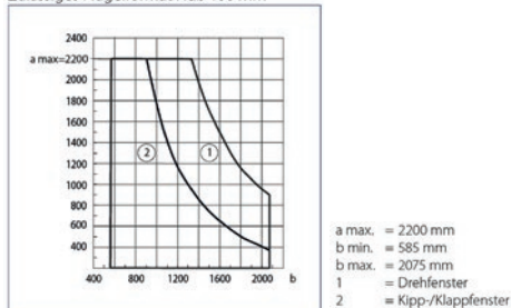
Zulässiges Flügelformat Hub 100 mm
