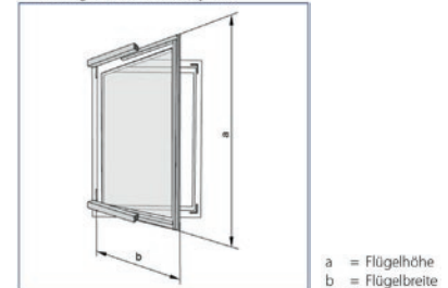
Ermittlung des Motorhubs Syncro
