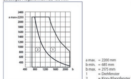
Zulässiges Flügelformat Hub 150 mm
